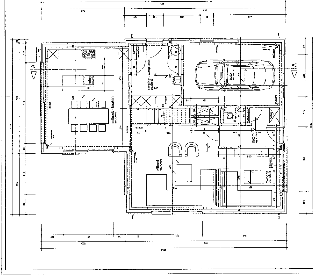
GELIJKLOERS 1/50
