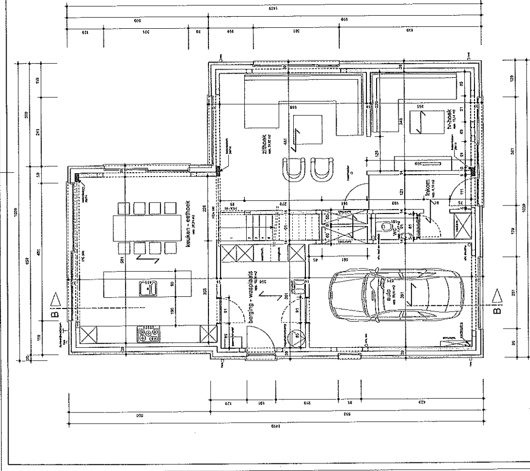
GELUKVLOERS 1/50
